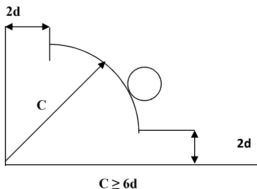
Rysunek 7: Wzajemne usytuowanie otworu i naroża szyb
