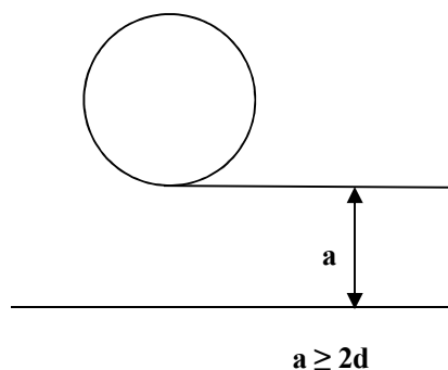
Rysunek 5: Wzajemne usytuowanie otworu i obrzeża szyb
