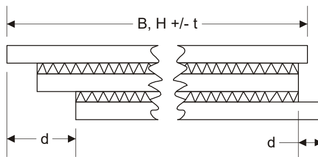
Rys. 14 –przemieszczenia tafli w szkle warstwowym
