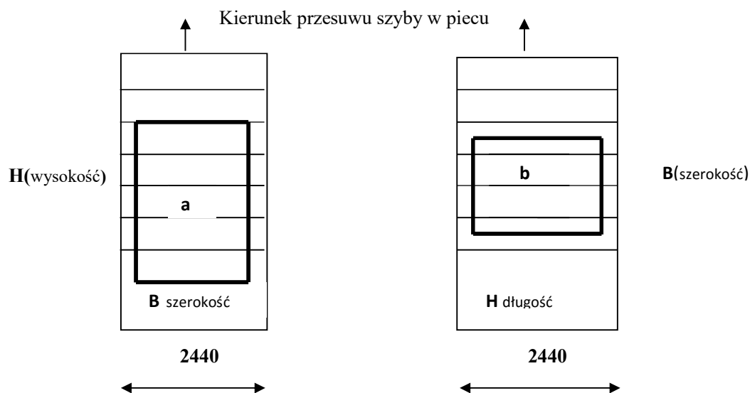
Rysunek 10: Hartowanie kierunkowe
