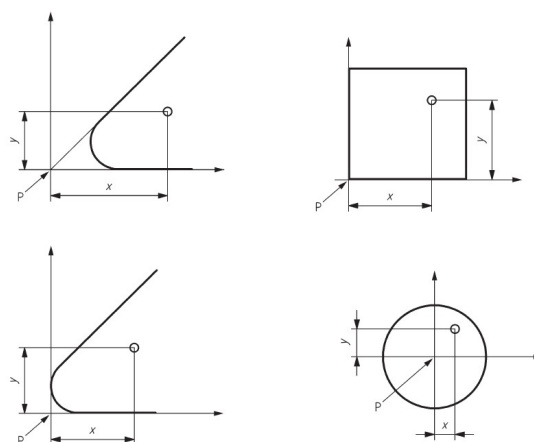
Rysunek 9: Przykłady rozmieszczenia otworów w zależności od punktu odniesienia
