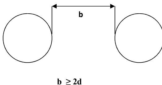
Rysunek 6: Wzajemne usytuowanie dwóch otworów
