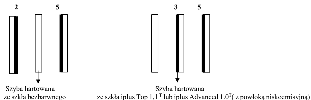
Rysunek 21: Schemat zastosowania szkła hartowanego w szybie dwukomorowej
