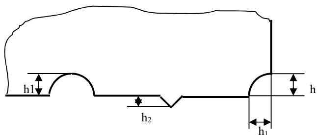
Rysunek 2: Szczerby i naddatki – widok powierzchni
